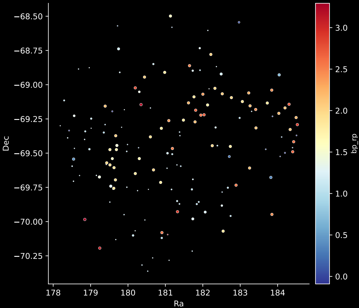
APOGEE DR17 Field: [280-33-O] Stars: 158
