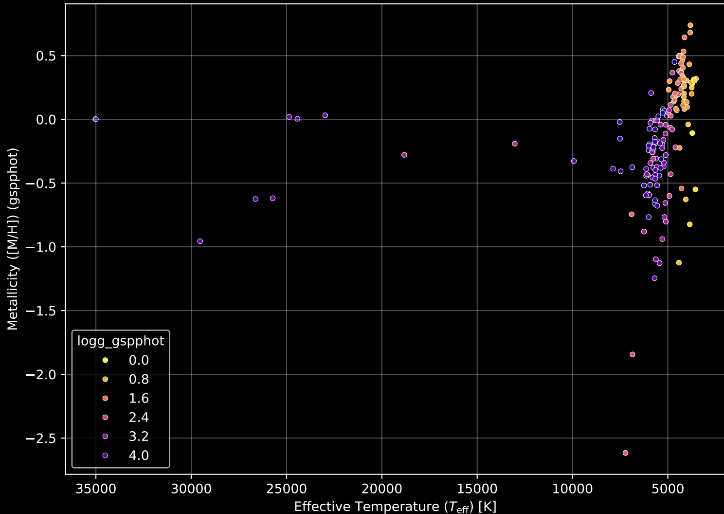
APOGEE DR17 Field: [280-33-O] Stellar Population Parameters (n= 158)
