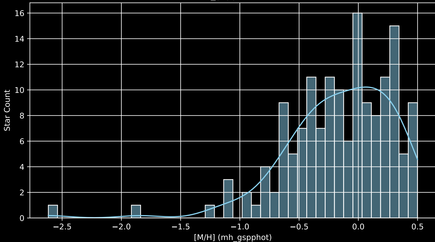
APOGEE DR17 Field: [280-33-O [M/H] (mh_gspphot) (n= 154)
